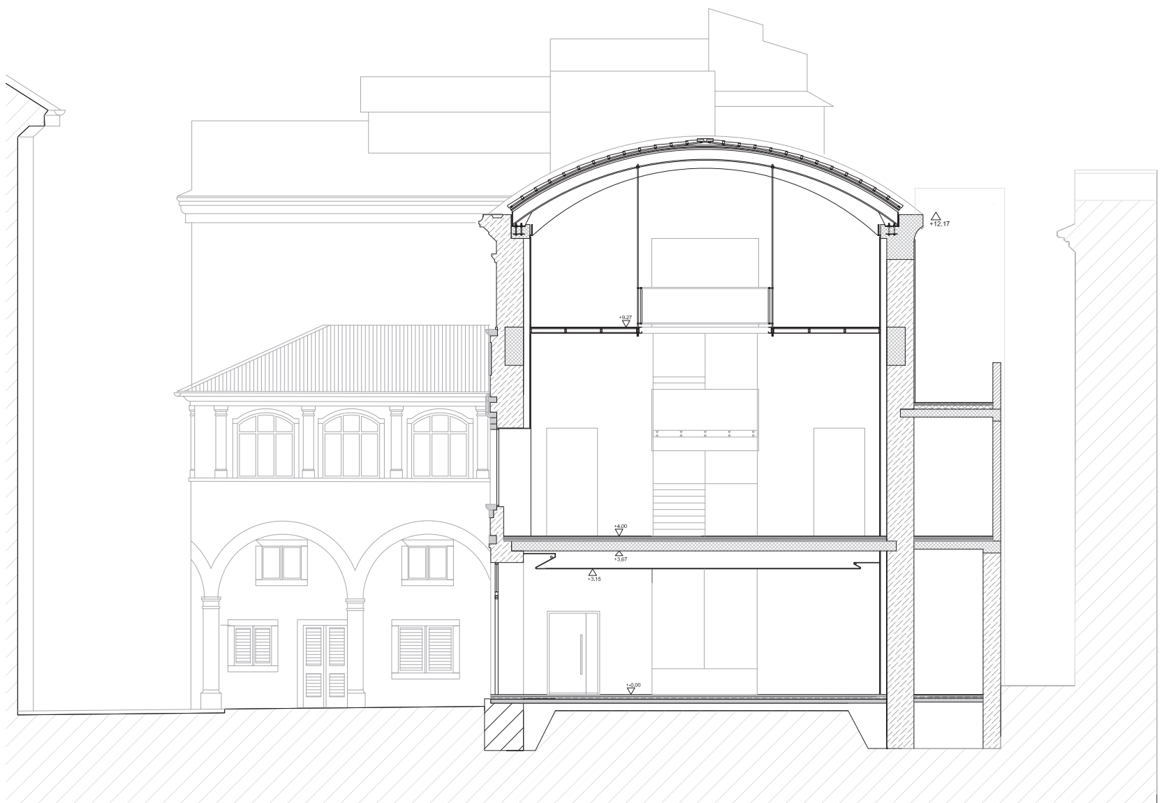
prečni prerez
