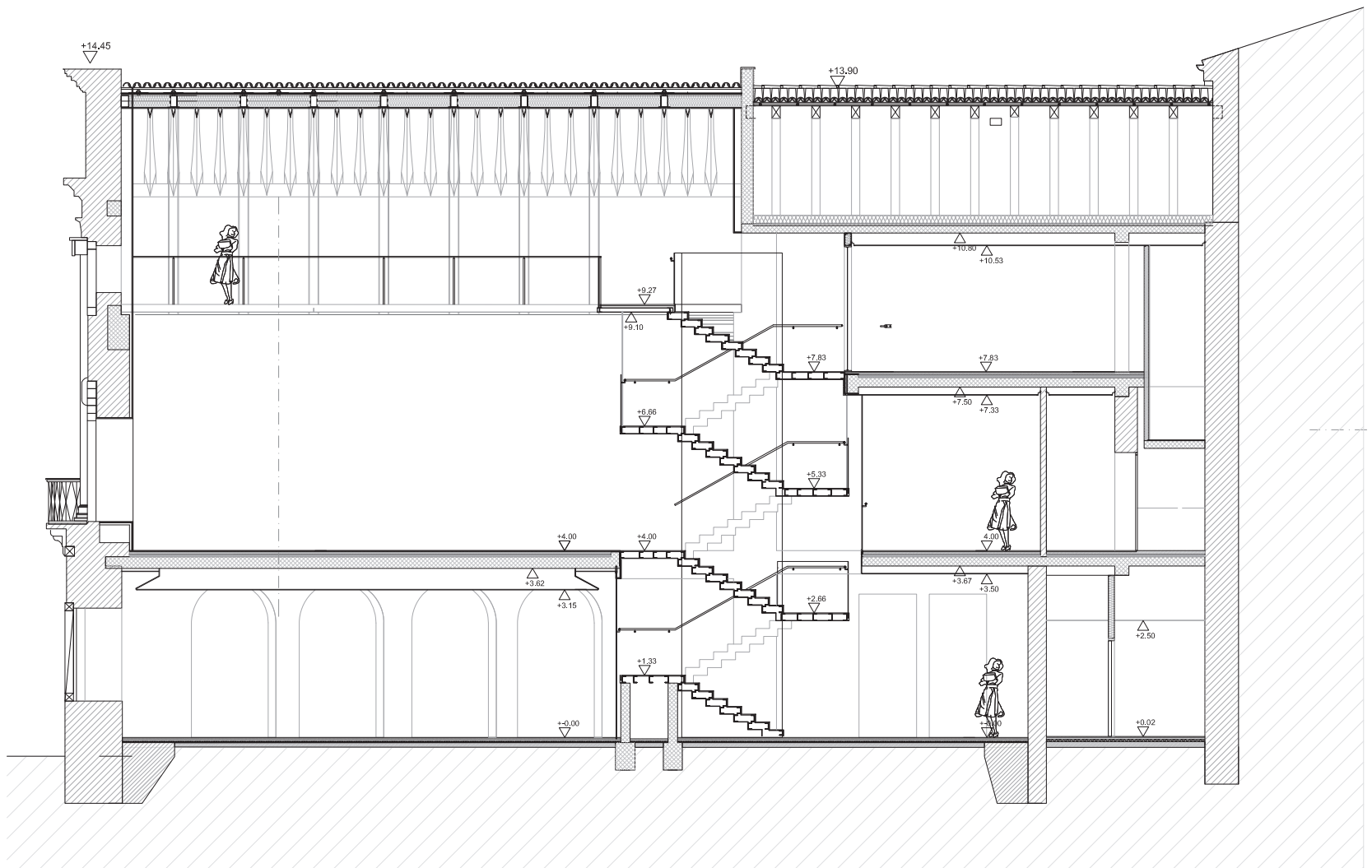
vzdolzni prerez
